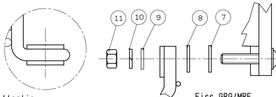
Dettaglio: Piedini di appoggio griglia
