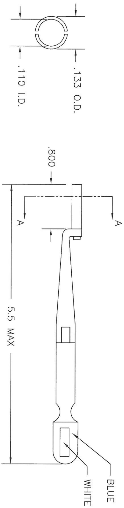
VIEW A-A
