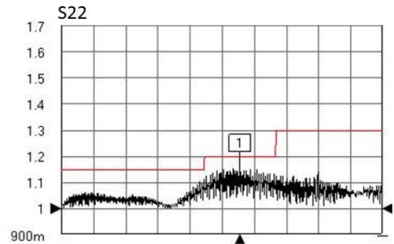
PE3TC0201-24 VSWR
