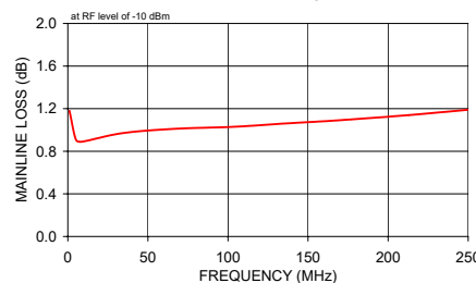
ZDC-10-1-75+ MAINLINE LOSS
