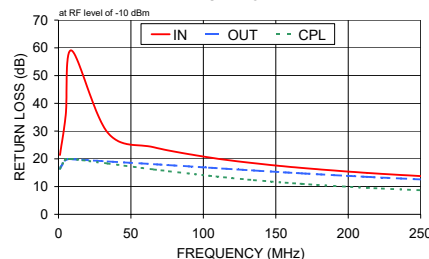
ZDC-10-1-75+ RETURN LOSS
